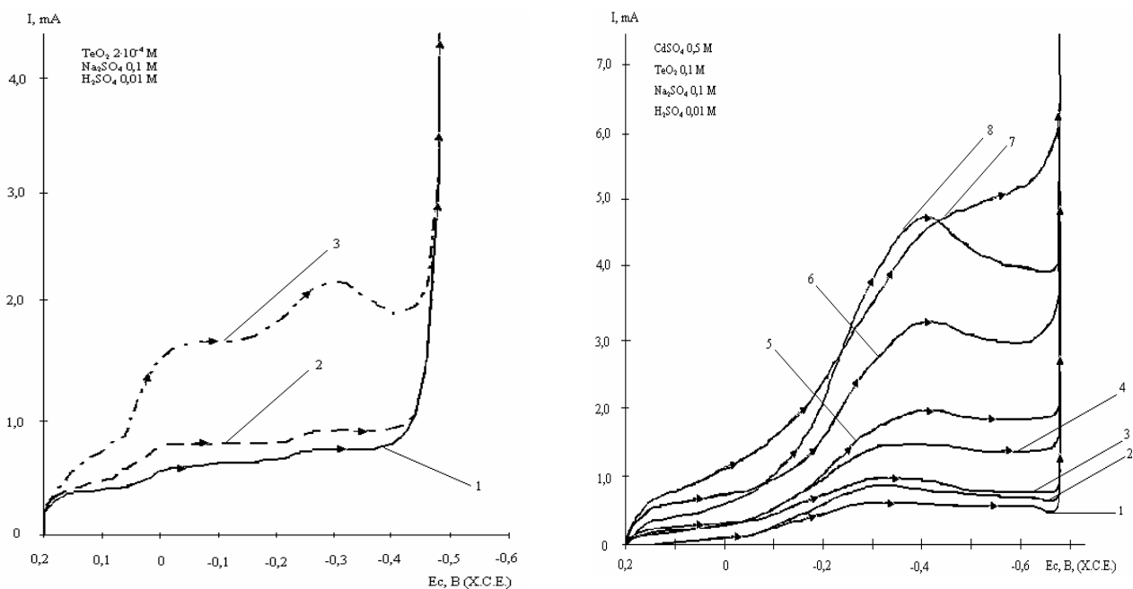
Рис. 5. Хроновольтамперограми на підкладках TiN в розчині, відповідному електроліту для осадження CdTe при швидкостях розгортки катодного потенціалу мВ/с: 1 – 5; 2 – 10; 3 – 20; 4 – 50; 5 – 100; 6 – 200; 7 – 500; 8 – 200 за умов перемішування електроліту.
