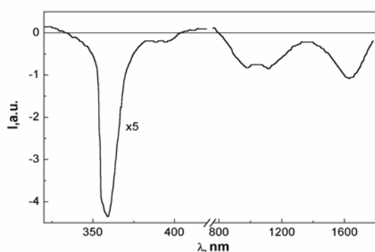
Рис. 4. Спектральна чутливість електретного стану кристалу \text{CdI}_2 , попередньо опроміненого в атмосфері повітря при 295 К інтегральним світлом від ксенонової лампи протягом 10 хв і охолодженого до 90 К.
