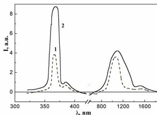
Рис. 3 Спектральна чутливість електретного стану кристалу CdI_2 , охолодженого від 295 до 90 К у присутності зовнішнього електричного поля величиною 2 \cdot 10^3 В/см (1) і -2 \cdot 10^3 В/см (2).
