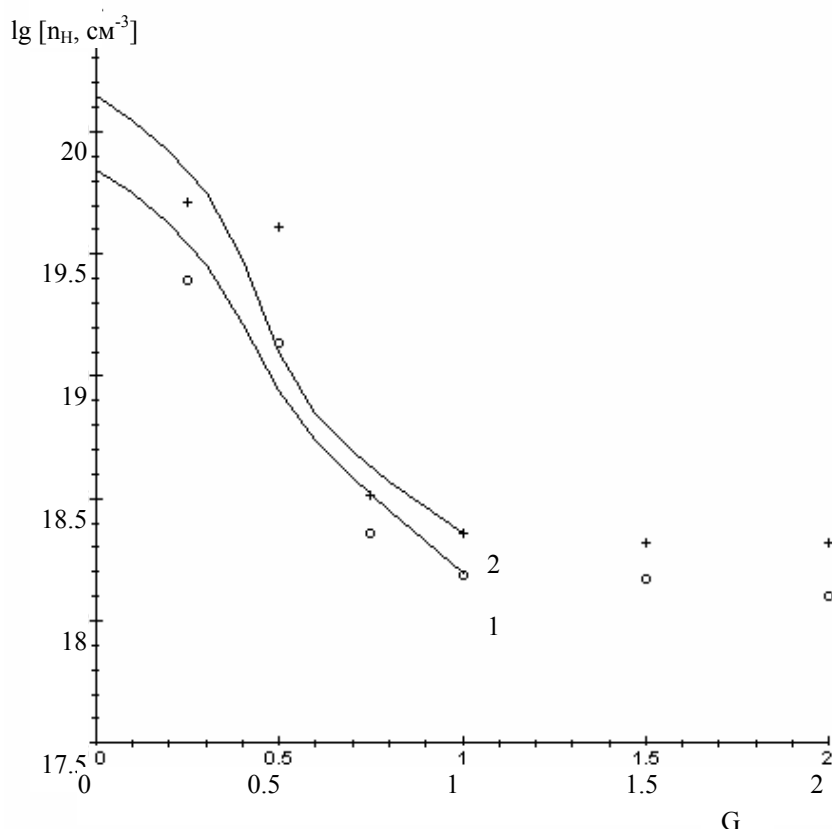
Рис. 1. Залежність концентрації носіїв струму у кристалах PbSe:Тl від концентрації надлишкового свинцю ( G=N_{Pb}/N_{Tl} ) для вмісту талію N_{Tl} , ат. %: 1 – 0,4; 2 – 0,8 (o, + – експеримент; – – розрахунок).
