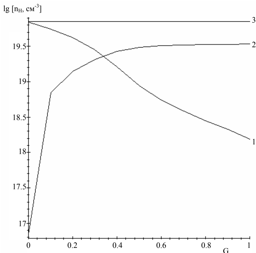
Рис. 2. Теоретичні залежності холлівської концентрації (1 – n_H ), концентрації вакансій селену (2 – (V_{Se}^{2+}) ) та міжвузлового талію (3 – (Tl_i^-) ) у PbSe:Tl від вмісту свинцю ( G=N_{Pb}/N_{Tl} ). Вміст талію N_{Tl}=0,4 ат. %.
