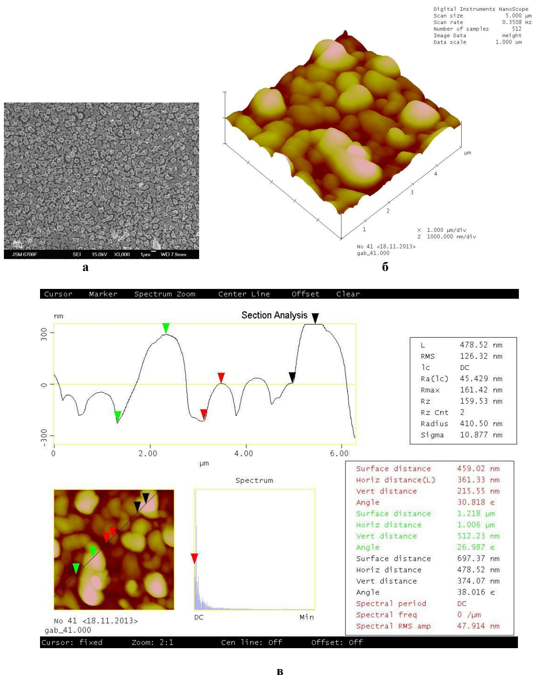
Рис. 7. Плівка нікелю завтовшки 100 нм на лейкосапфірі відпалена при 1200 °С протягом 2 хв у вакуумі: а – вигляд плівки під скануючим мікроскопом, x3000; б – вигляд плівки під атомно-силовим мікроскопом; в – профілограма плівки.
