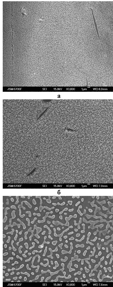
Рис. 1. Плівка металу завтовшки 100 нм на оксидних матеріалах відпалена при 1000 °С у вакуумі, x3000: а – хром на кварцовому склі, відпал 20 хв; б – нікель на кварцовому склі, відпал 2 хв; в – нікель на алюмооксидній кераміці відпал 20 хв.
