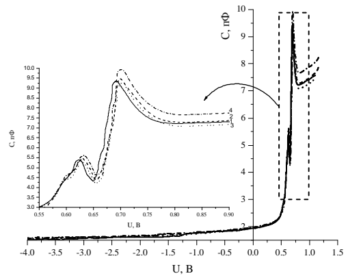
Рис. 5. Зміна вольт-фарадних характеристик сенсора (перехід емітер-база) після впливу магнітного поля. 1 – вихідна крива; 2 – після витримки протягом 5 год; 3 – після витримки протягом 10 год; 4 – після витримки протягом 15 год.
