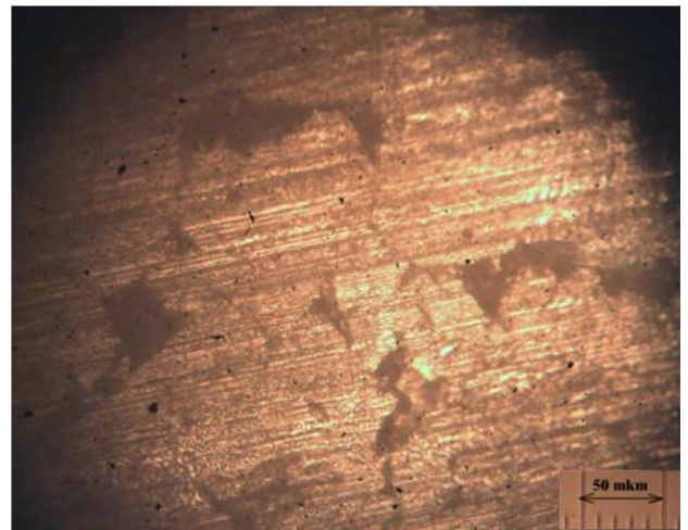
Рис. 3. Мікрофотографії пресованих брикетів Pb_{49.75}Te_{50.00}:Sb_{0.25} .
